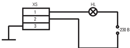
XS - розетка генератора; HL - лампа 25 Вт
